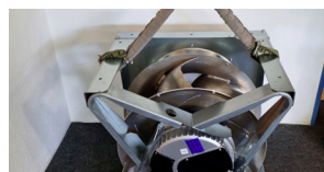
Structure porteuse
