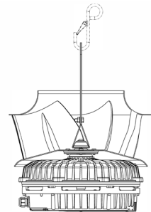
1. Hebehilfe – 2. Sicherungsschraube – 3. Sicherungsmutter
