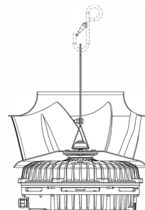
1. Sangle de manutention 2. Vis de serrage 3. Ecrus de serrage
