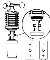
Wind Sensor LTV-W2
