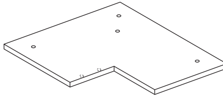
B 485*485*12mm(1pc)
