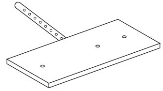
C 485*205*12mm(1pc)
