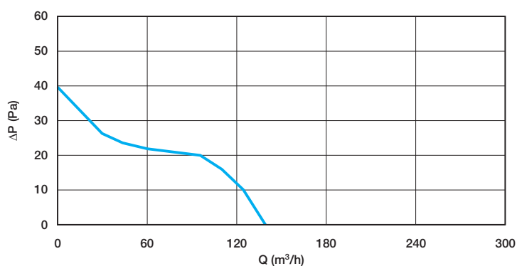
Courbe aérodynamique GRAPHIC 125
