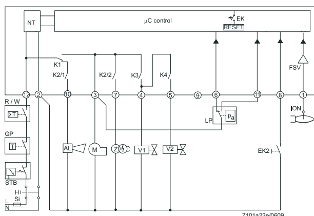
Schéma interne et déroulement du programme LME21...
