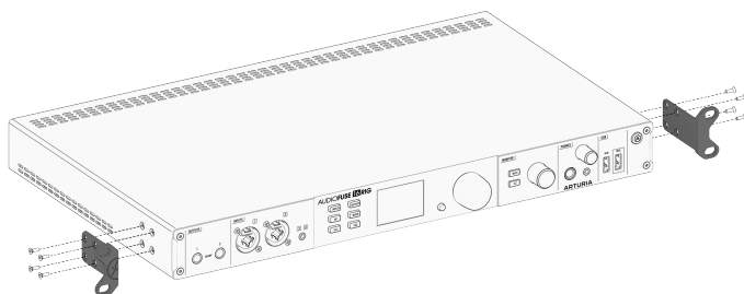
AudioFuse 16Rig ラックマウント取付図
