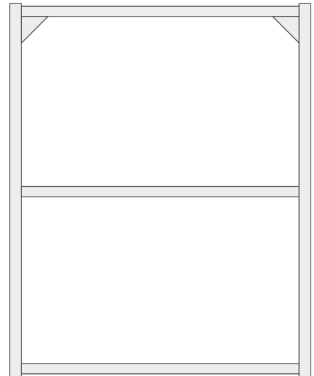
Bovenkastelement met planken H 75 cm verkrijgbaar in 40×15 cm 40×30 cm 60×15 cm 60×30 cm
