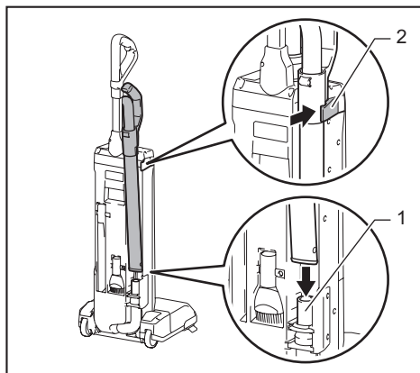
► 1. Joint 2. Pipe holder
