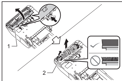
► 1. Bottom plate 2. Brushroll
