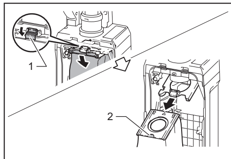
► 1. Seguro 2. Tira
