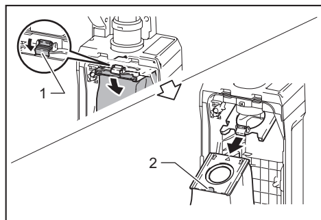
► 1. Latch 2. Strip
