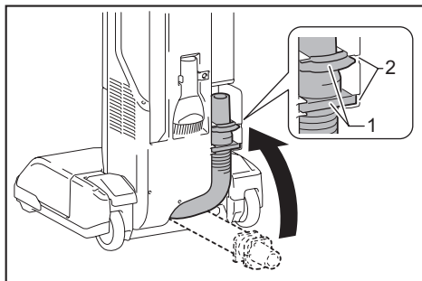
► 1. Lengüeta 2. Ranura
