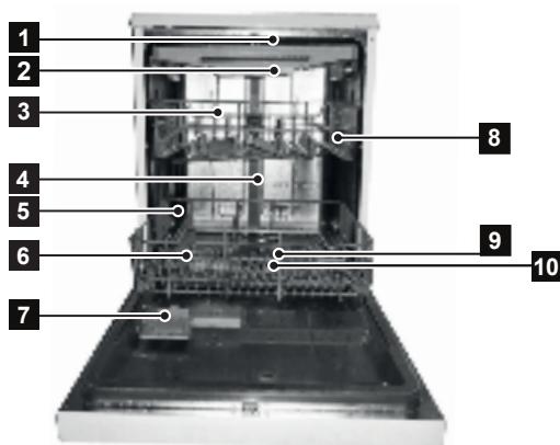
Čelní pohled
