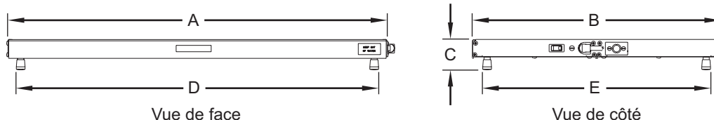
Dimensions — Modèles GRS
