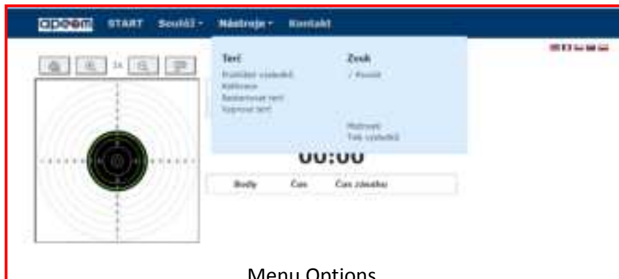
Menu Options
