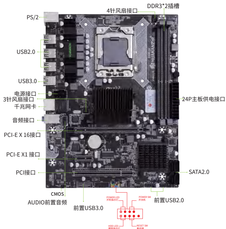
图1-1 X58-RX3.0主板图解
