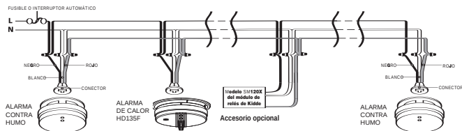
FIGURA 4. DIAGRAMA DE CABLEADO DE INTERCONEXIÓN
