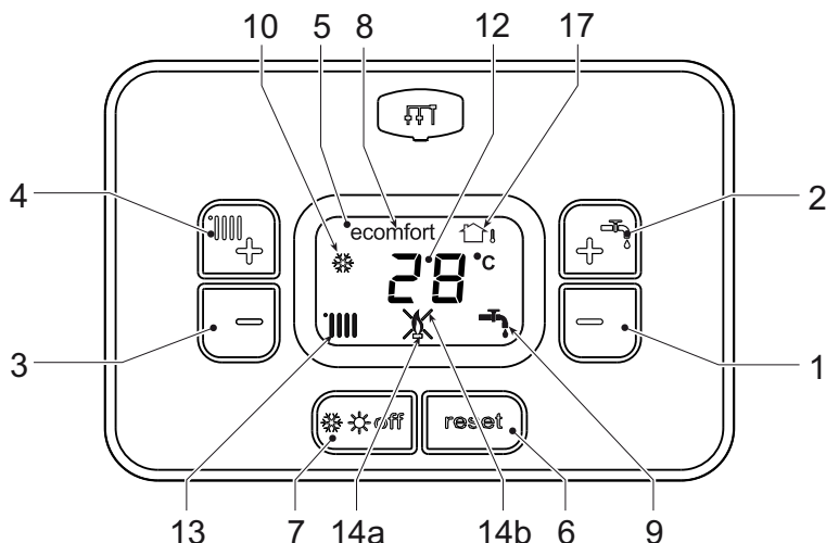
fig. 1- Panoul de control
