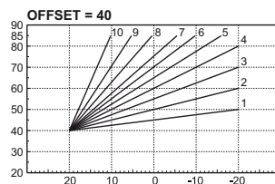
fig. 15- Exemplet de deplasare paralelă a curbelor de compensare
