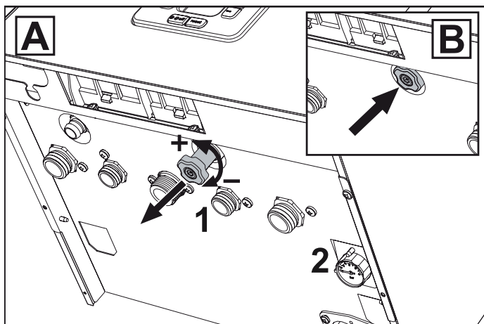
wygląd 16- Pokrętko napełniania
