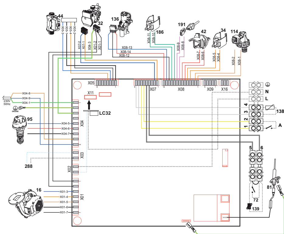
fig. 40- Esquema eléctrico
