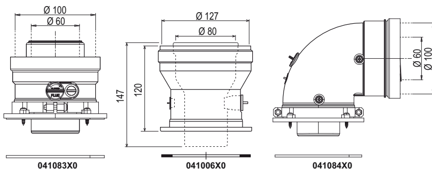
εικ. 21- Εξαρτήματα σύνδεσης για ομοαξονικούς αγωγούς
