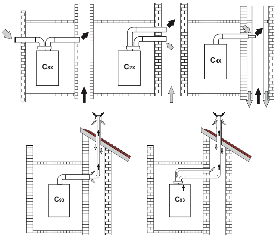
εικ. 26 Παραδείγματα σύνδεσης σε καπνοδόχους (⇨ = Αέρας / ⇨ = Καυσάστρια)
