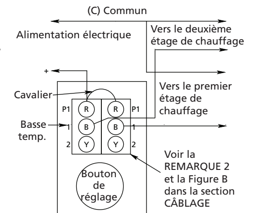
Figure 7 – Thermostats SPDT/SPDT contrôlant un système de chauffage à deux étages
