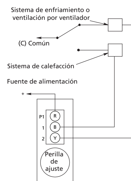
Figura 3 – Termostatos SPDT/SPDT en Control de Sistemas de Calefacción o Ventilación
