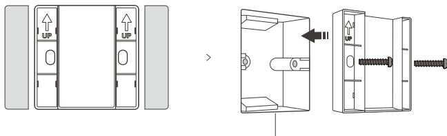
Монтажная коробка тип 86
