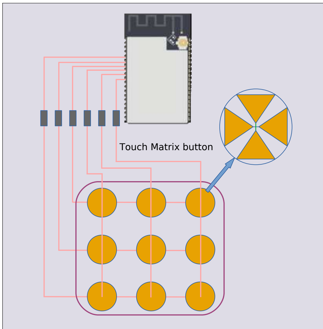
图 28: 触摸矩阵
