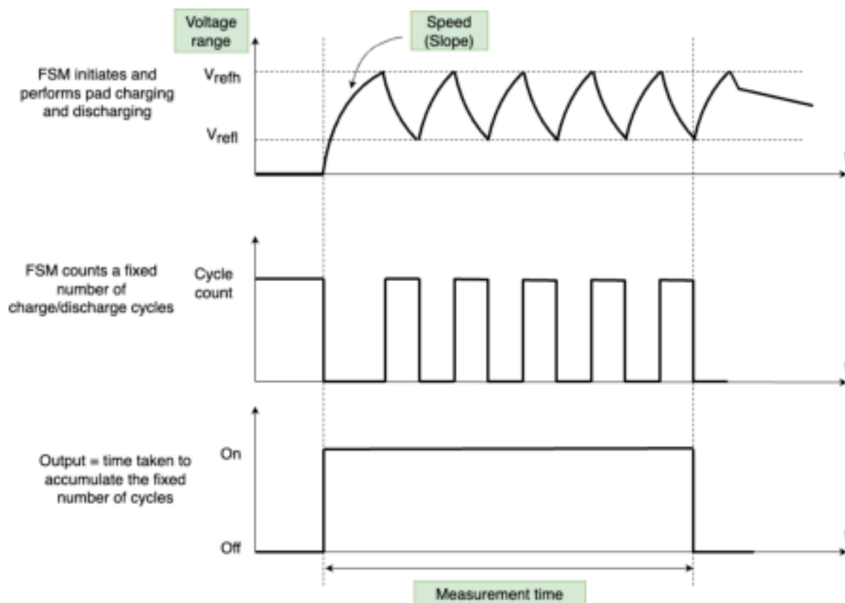
图 21: 触摸传感器 - 测量参数之间的关系
