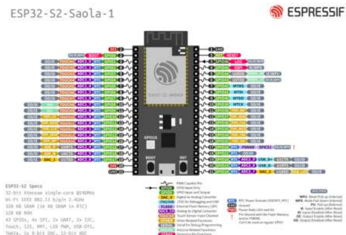
图 4: ESP32-S2-Saola-1 管脚布局 (点击放大)
