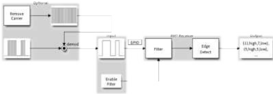
图 16: RMT 接收器概述
