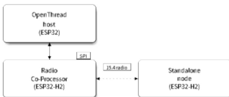
图 43: OpenThread 设备模式
