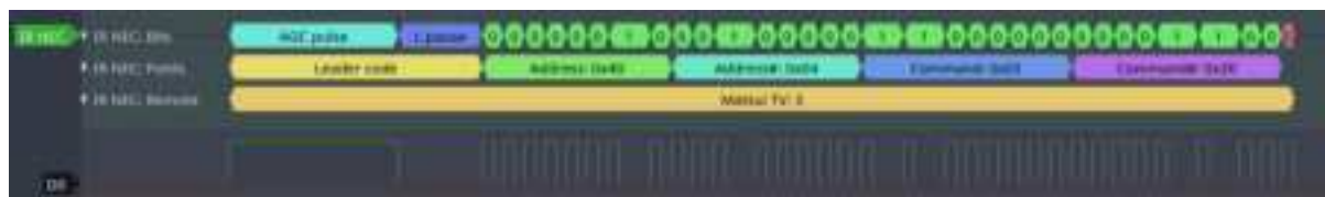
图 19: 红外 NEC 帧
