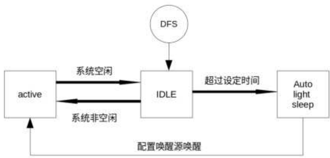
图 65: Auto Light-sleep 模式工作流程图
