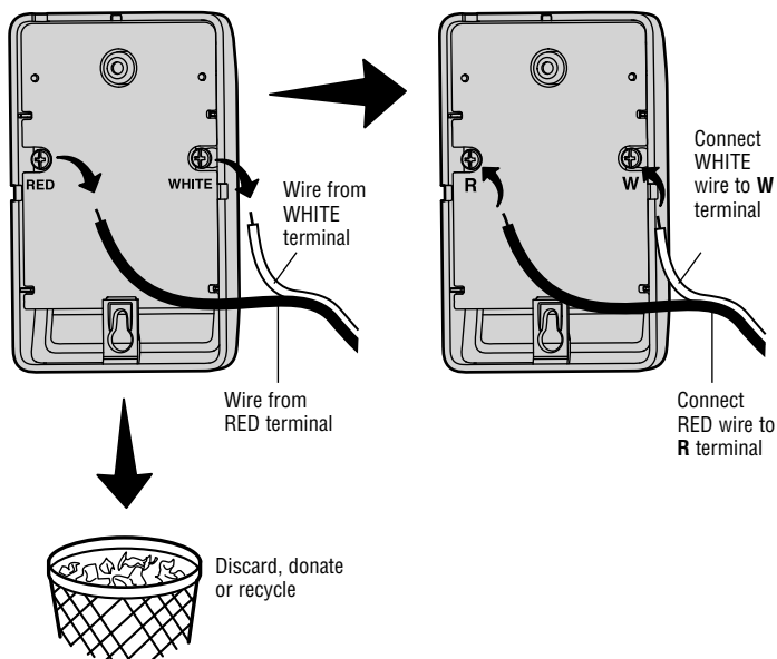
Existing Door Control
