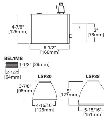
LZR510 PAR LAMP METAL HALIDE LAMPHOLDER
