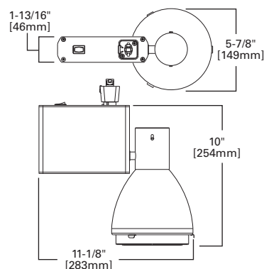
LZR510 ED17 PAR LAMP METAL HALIDE LAMPHOLDER
