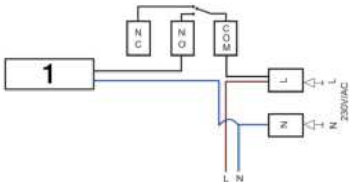
1) Elektrický ohřívač / Tepelný pohon
