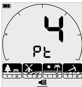
Экран настройки порога высоты сигнала.
