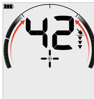
Слабый/смещенный от центра сигнал цели: включено меньше сегментов распознавания. Цель расположена ближе к внешней стороне катушки.
