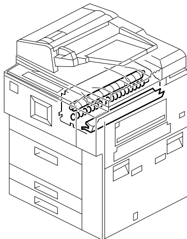
37. PCU 3
