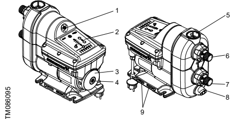
مضخة SCALA2 من جرونفويس
