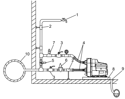
تقوية ضغط أنبوب الماء الرئيسي، مضخة SCALA2
