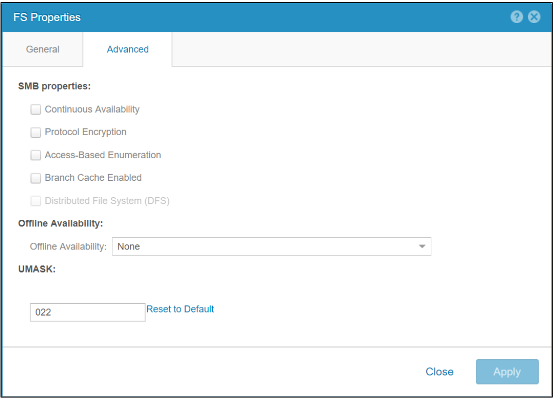
Figure 34 UMASK
