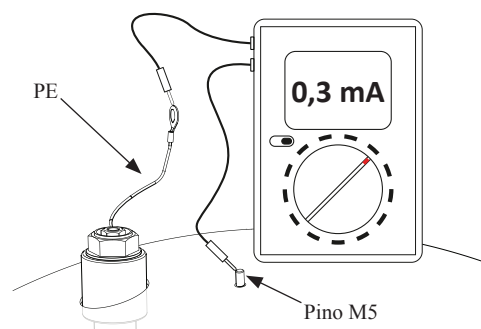
Medição da intensidade de corrente contínua de proteção
