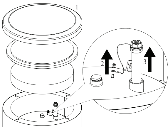
Substituição do ânodo de magnésio protetor
