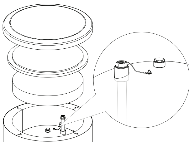
Ânodo de magnésio protetor isolado
