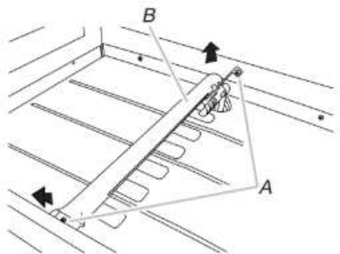
A. Tornillos B. Quemador para hornear
