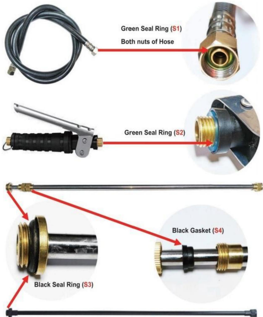
Anillo de sello verde (S1) 9X13X2(Instalado)
