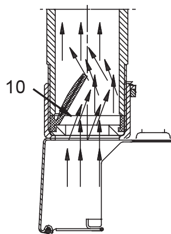
Rys. 58 Zawór zwrotny w króciec tłoczny pompy Unilift
