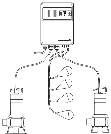
Rys. 49 Pompy Unilift AP35B/AP50B z sterownikiem poziom LCD
