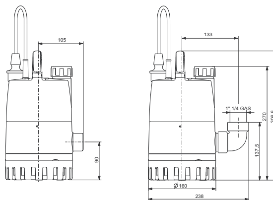
Rys. 5 Wymiary pompy
