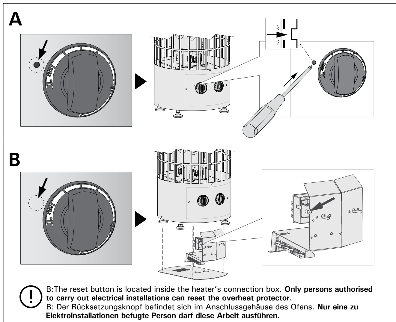
Figure 10. Reset button for overheat protector Abbildung 10. Rücksetzkopf des Überhitzungsschutzes
