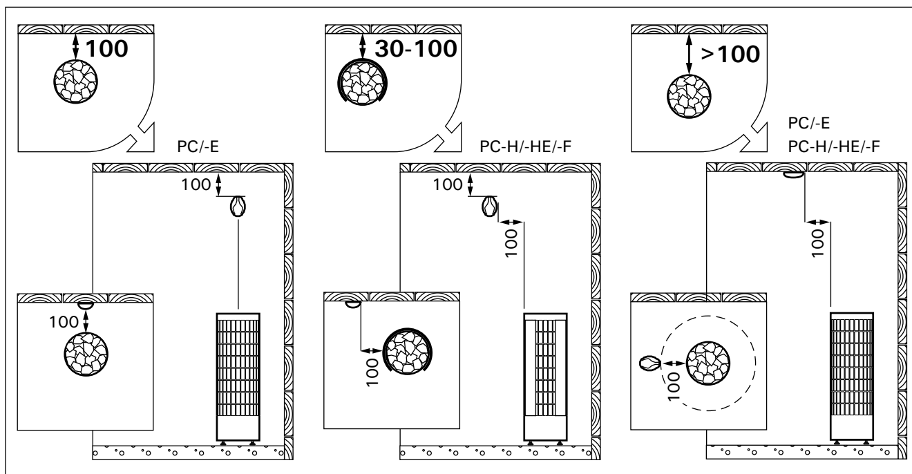
Kuva 8. Anturin asentaminen (mitat millimetreinä) Bild 8. Montering av qivaren (måttan i millimeter)
