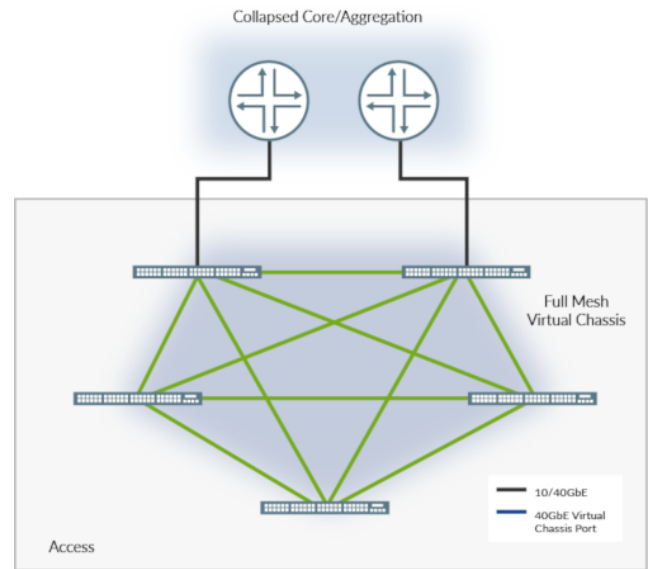
그림 3: 데이터센터에서 전체 메시/Virtual Chassis를 사용하여 구성된 EX4300 스위치입니다.
