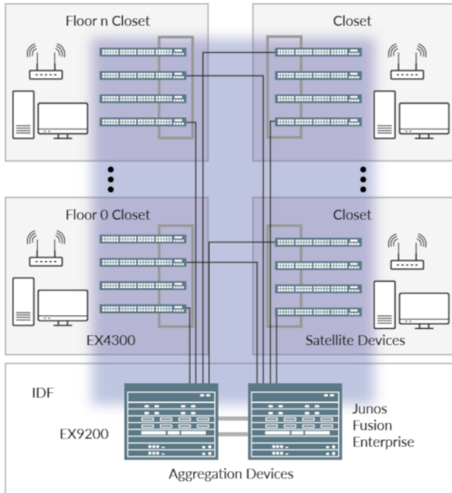
그림 5: Junos Fusion Enterprise 아키텍처에서 위성 디바이스로 작동하는 EX4300 스위치.
