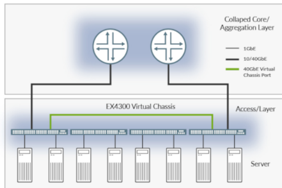
그림 2: Virtual Chassis 기술이 적용된 EX4300 이더넷 스위치는 성능, 확장성 및 안정성이 뛰어난 데이터센터용 솔루션을 제공합니다.
