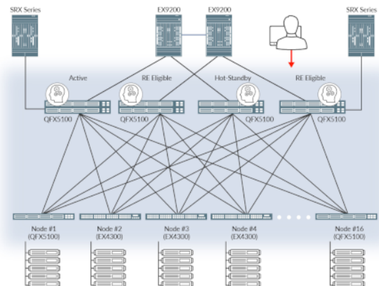
그림 4: Virtual Chassis Fabric 구성 내 액세스 계층의 EX4300, QFX3500, QFX3600 및 QFX5100.
