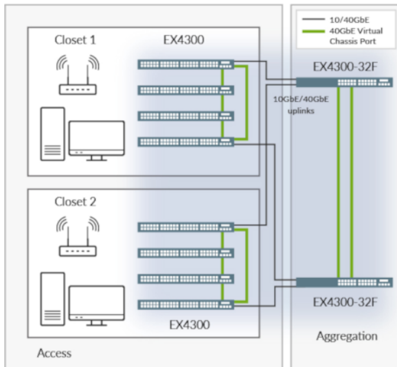
그림 1: Virtual Chassis 기술을 사용함으로써 최대 10개의 EX4300 스위치를 상호 연결해 건물 전체에 걸쳐 단일 논리적 디바이스를 구축할 수 있습니다.
