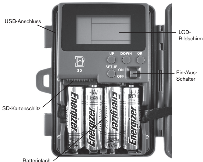
Bedienfeld (vorne geöffnet)
