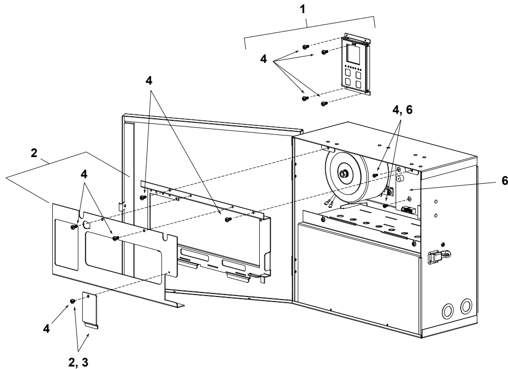
Figure 21c. Centro de control del AquaLink RS PureLink, 6613AP
