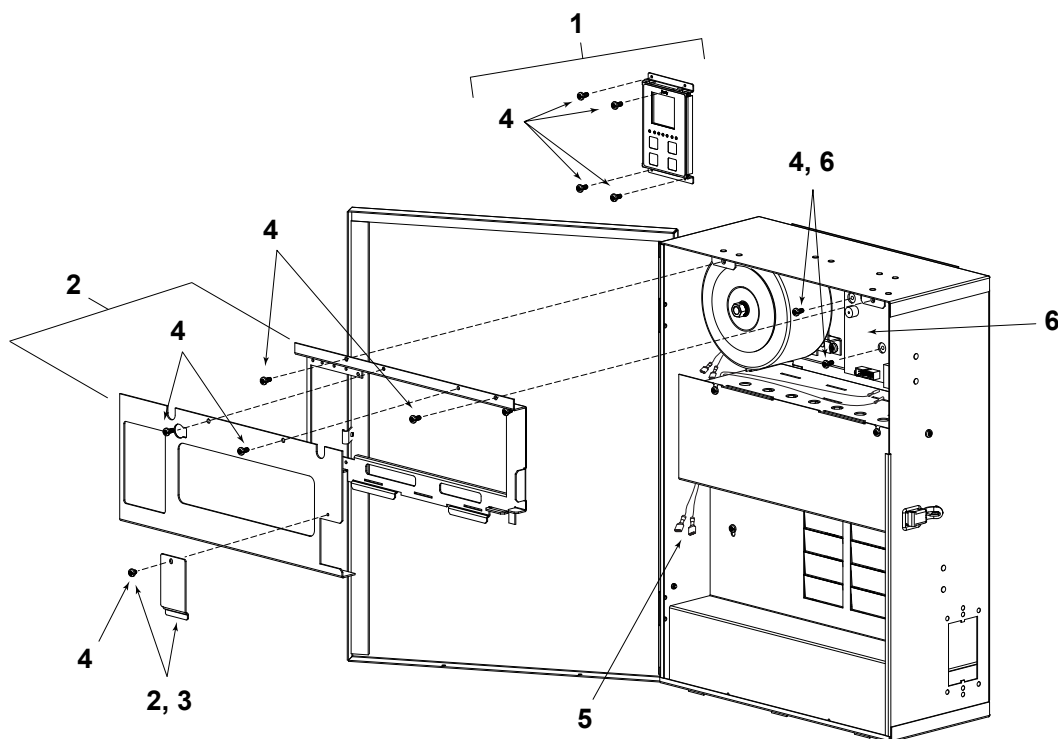
Figure 21b. Centro de control del AquaLink® RS PureLink™, 6614AP
