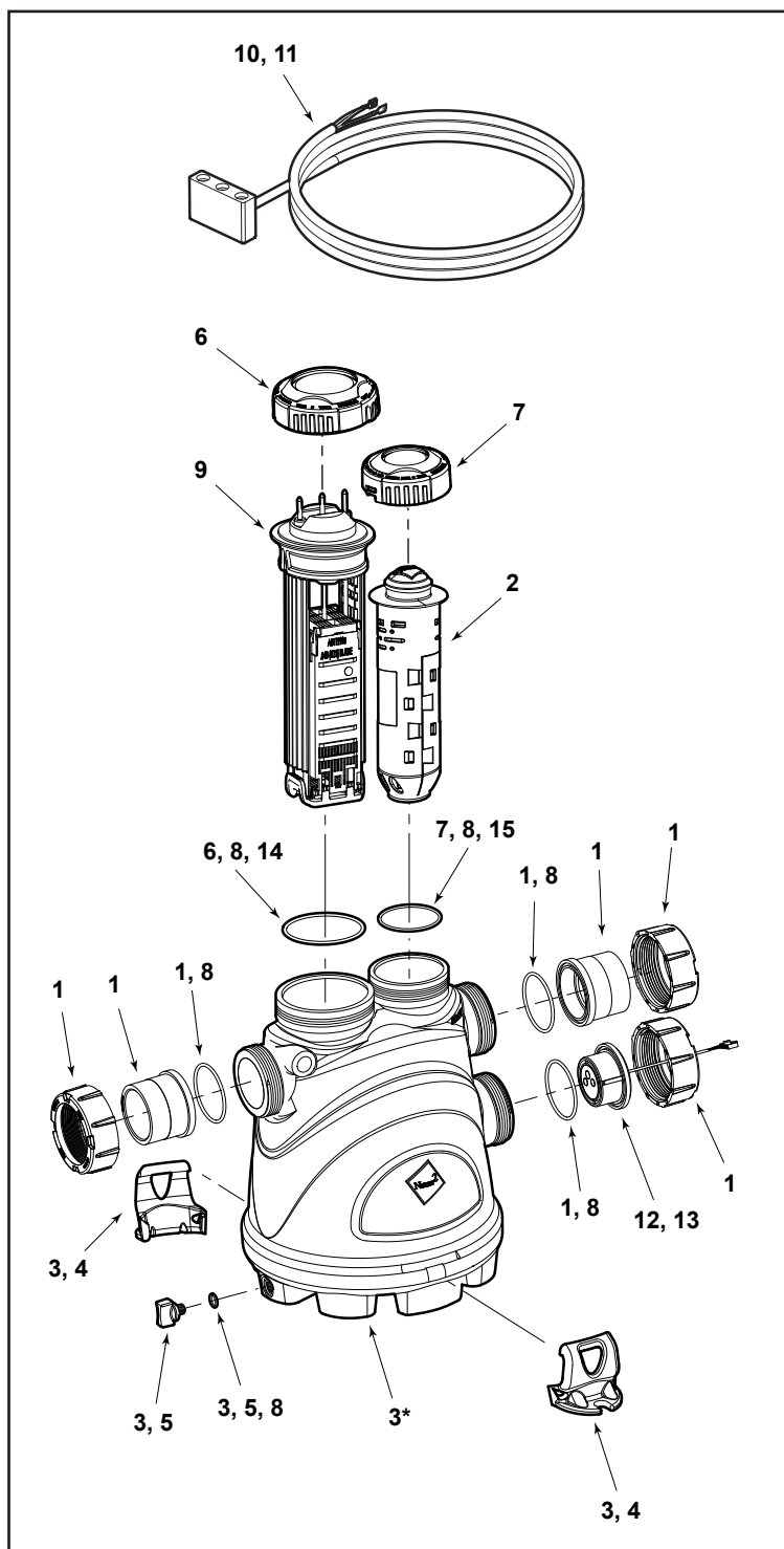
Figura 22. Vista ampliada del Nature 2 Fusion Soft
