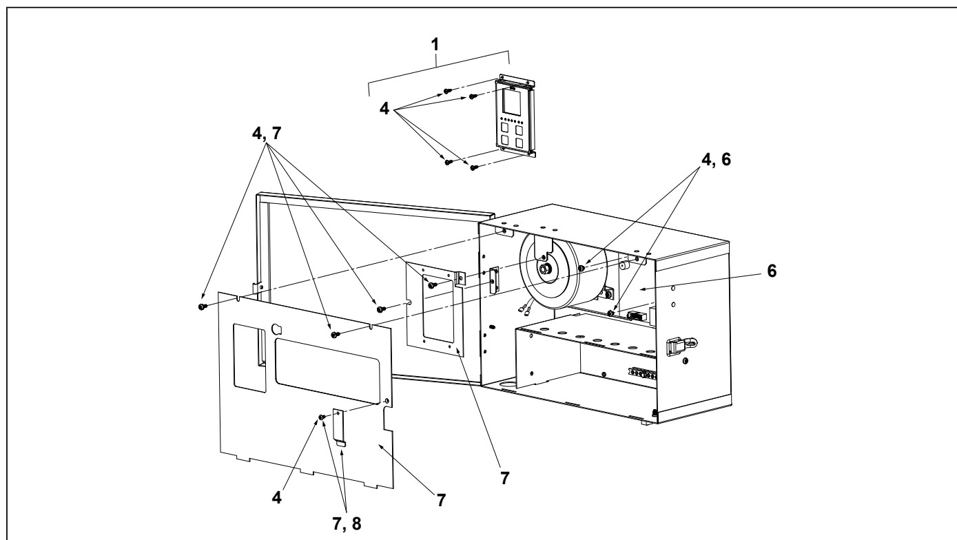
Figure 21a. Centro de alimentación del Nature 2 Fusion Soft
