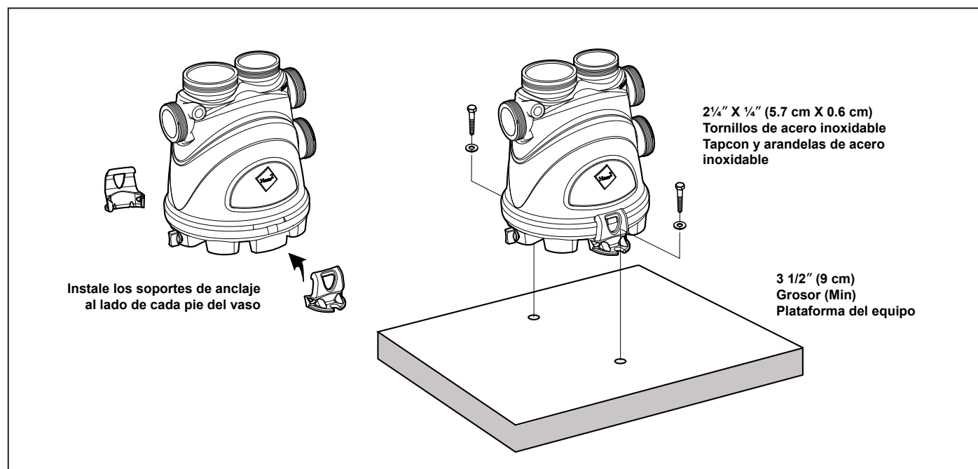
Figura 2. Instalación de los soportes de anclas
