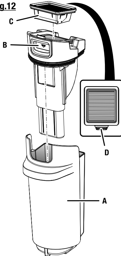
A - Dirty tank (réservoir d'eau sale, tanque sucio) B - Release button (bouton de dégagement, botón de liberación) C - Filter (filtre, filtro) D - Tab (languette, lengüeta)
