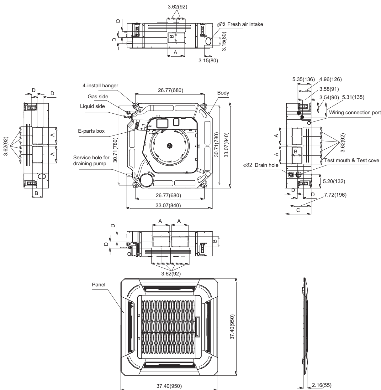
Fig. 5 — Indoor Unit (Sizes 24-48)
