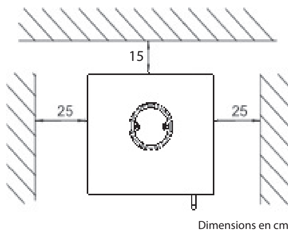
Poêle Installé droit dans le coin
