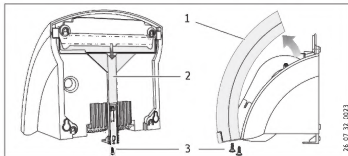
1 Házfedél 2 Tolózár 3 Csavarok
