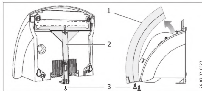
1 Kryt přístroje 2 Blokovací lišta 3 Šrouby
