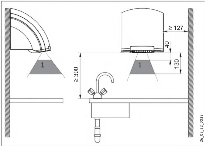
1 Erfassungsbereich der Infrarot-Näherungselektronik
