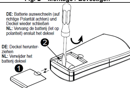
Fig. 3 – Batteriewechsel / Batterij vervangen
