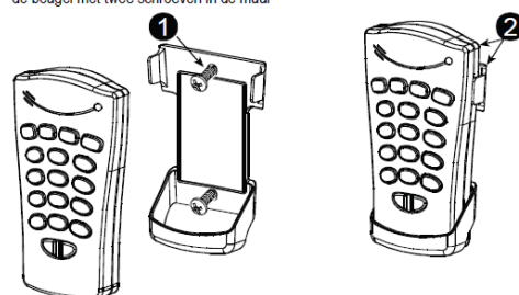
Fig. 2 – Montage / Bevestigen
