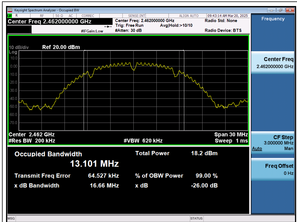
Test_Graph_802.11b_ANT1_2462_1Mbps_OBW
