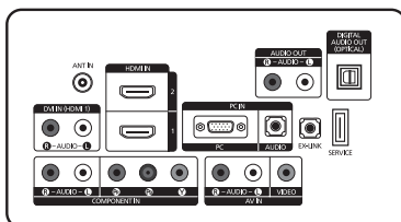
DETALLE DEL PANEL DE TERMINALES 5.2"H X 6.6"W
