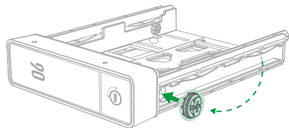
Montagestifte in die Montagelöcher befestigen
