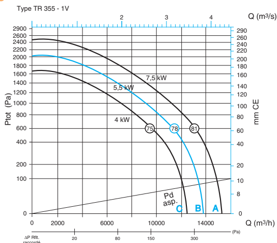
Caractéristiques aérodynamiques ProtectONE® TR 355 - 1V
