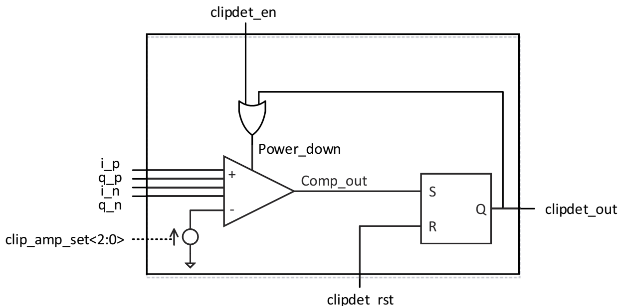
Fig 117. Clip detector 2
