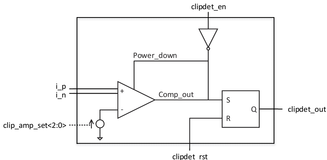
Fig 116. Clip detector 1
