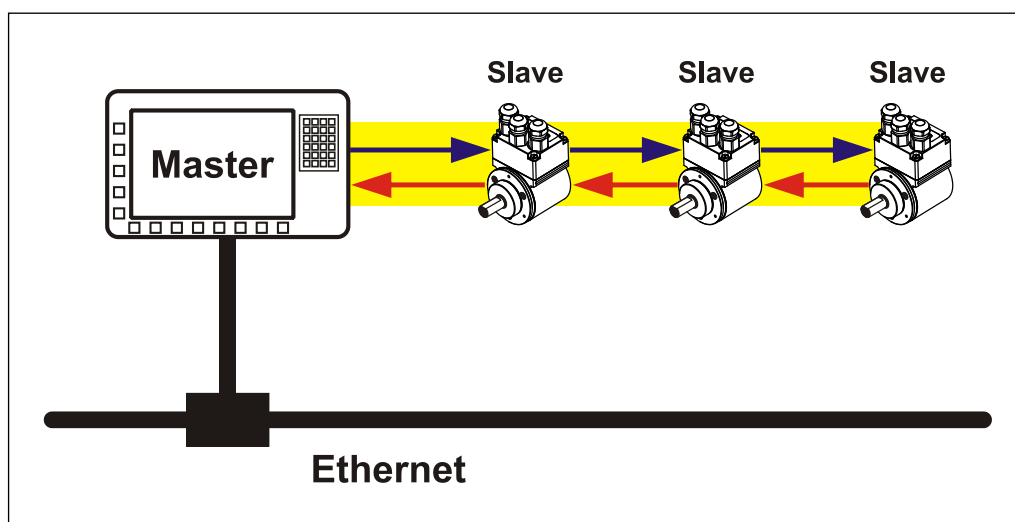
Abbildung 1: EtherCAT-Funktionsprinzip
