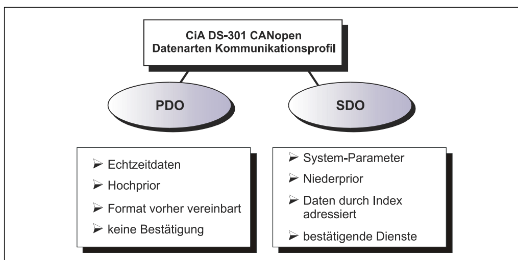
Abbildung 7: Gegenüberstellung von PDO/SDO-Eigenschaften
