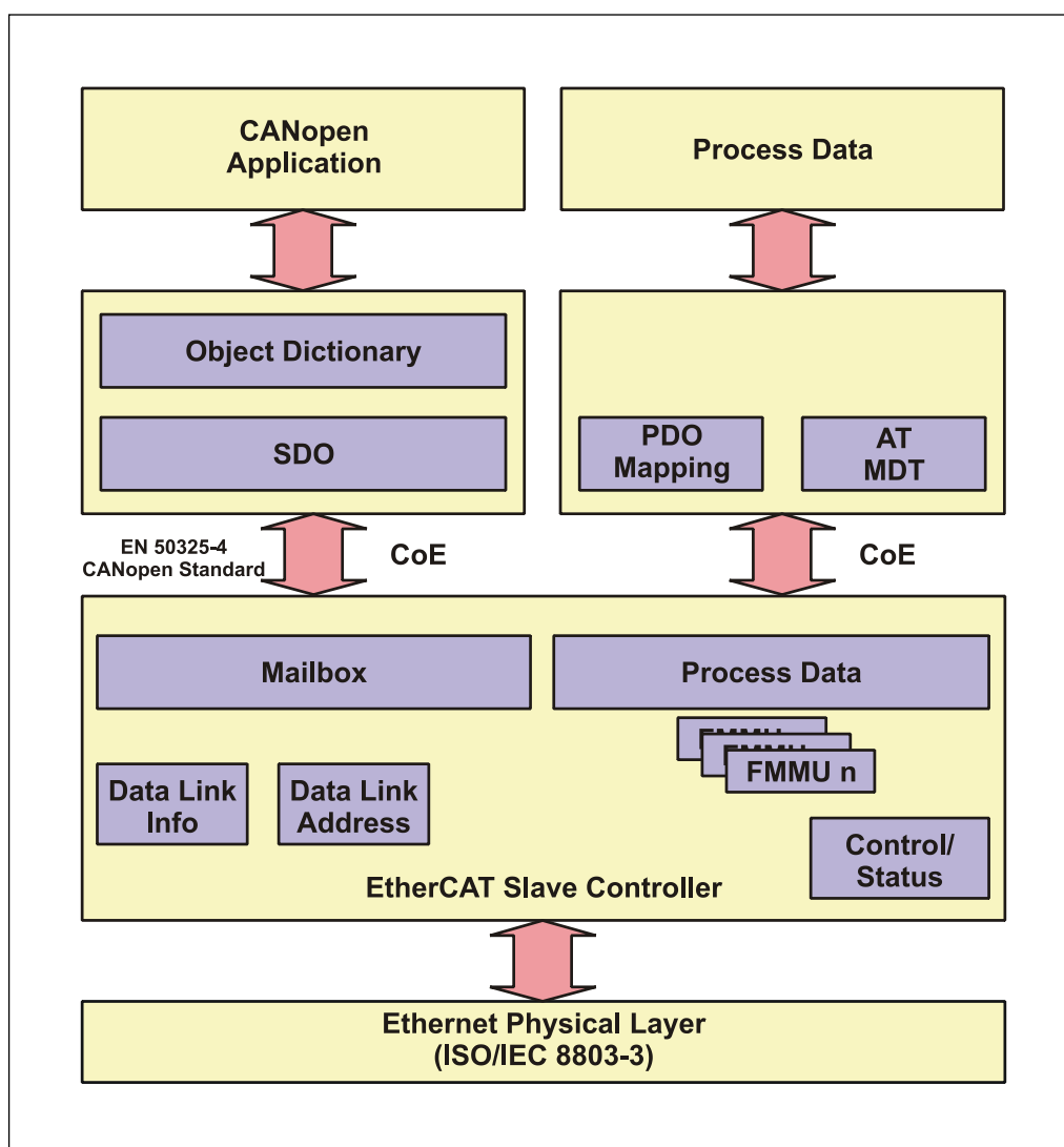
Abbildung 3: CANopen over EtherCAT Kommunikationsmechanismus
