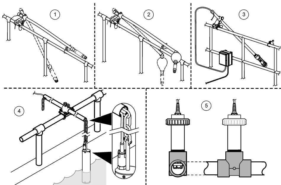
그림 5 설치 옵션
