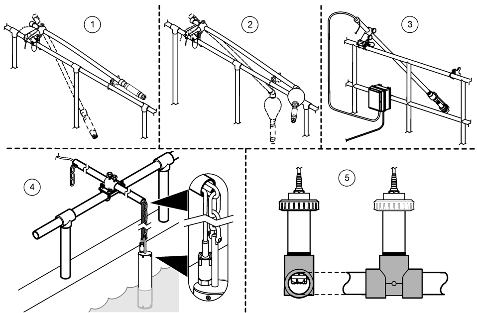
Figure 5 Options d'installation
