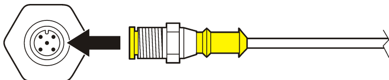
Figura 4 Conexión del sensor LDO (se muestra un sensor para ubicaciones no peligrosas)
