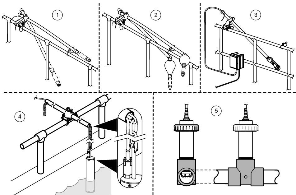
图 5 安装选项
