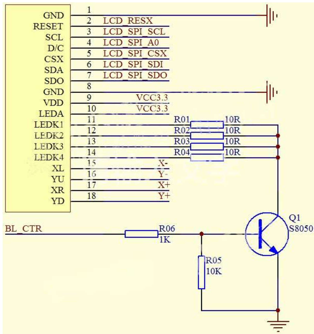
附图 6-1：显示屏 STP0320A2 4 线-SPI 串口参考应用电路
