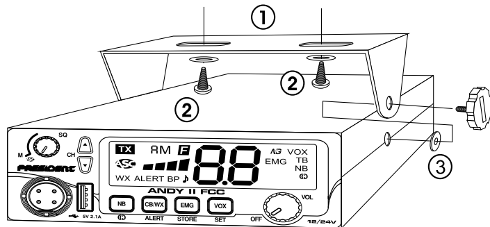
SCHEMA GÉNÉRAL DE MONTAGE
