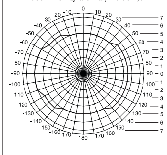
HF 360 - montaj la o înălțime de 2,8 m
