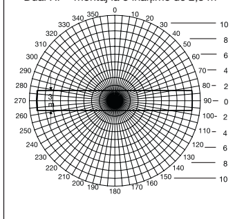
Dual HF - montaj la o înălțime de 2,8 m
