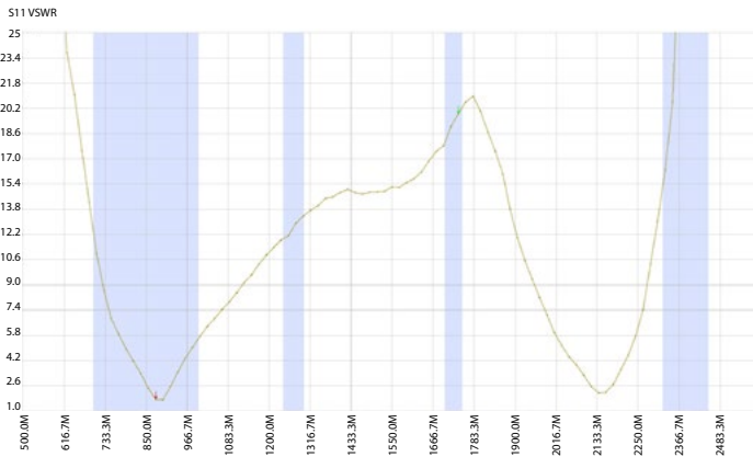
Gráfico de medición antena AN-I
