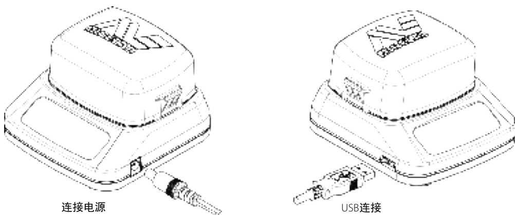
图 32 - BC10电源插头与USB接口
