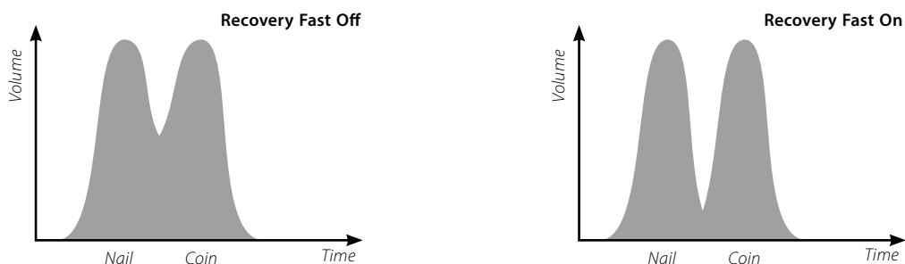
图 26 - 被混合的目标信号
