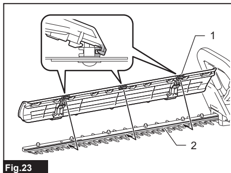
► 1. Claw 2. Groove
