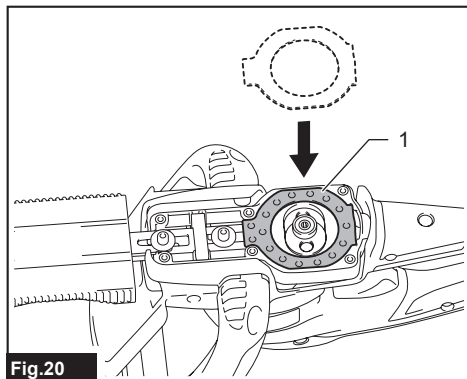
► 1. Plate
